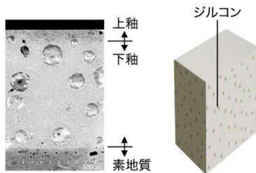
電子顕微鏡写真中の白色小斑点がジルコン鉱物
